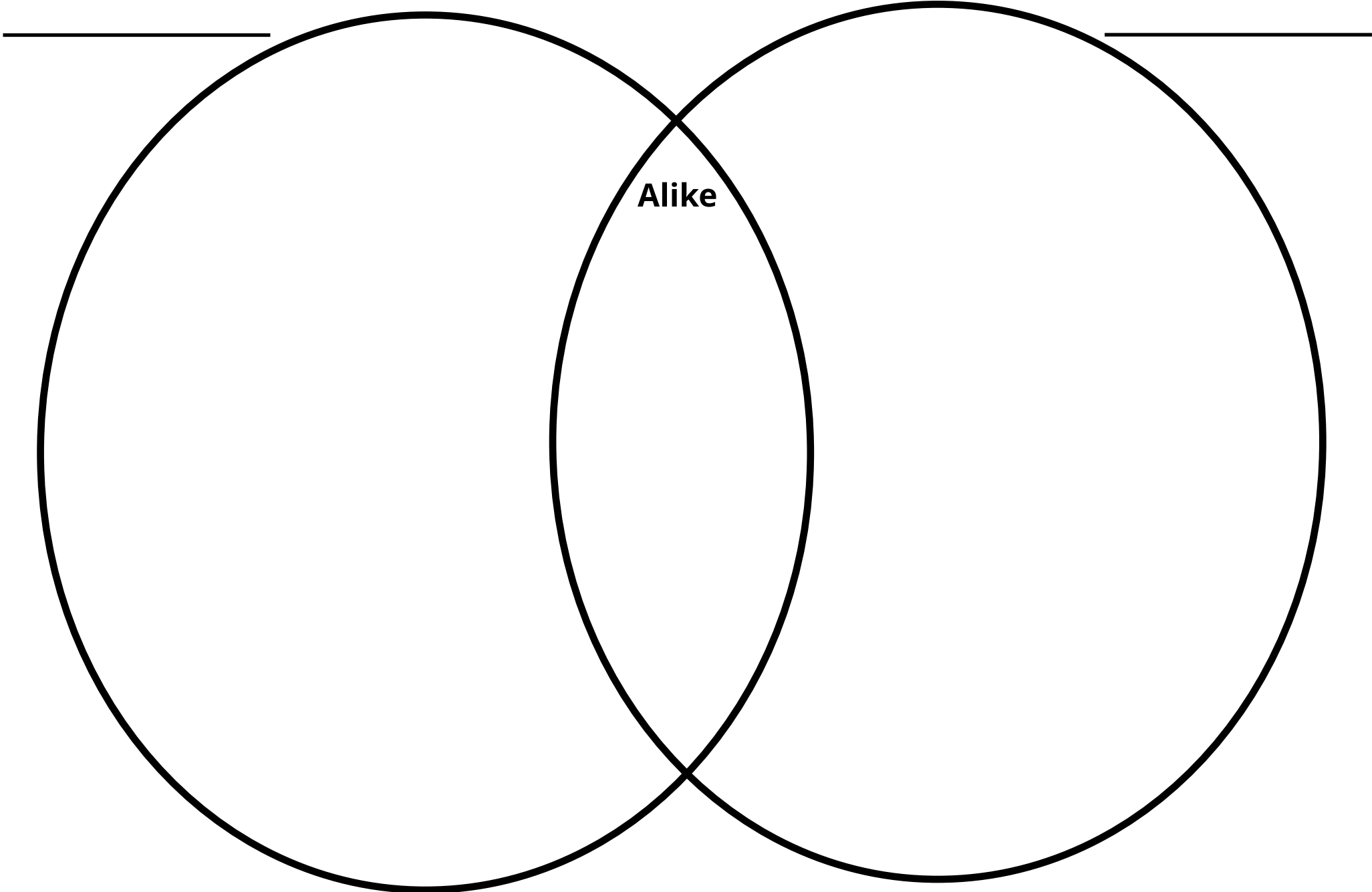
Venn Diagram
